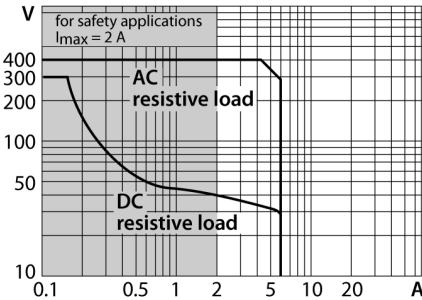
继电器输出-电流负载阈值曲线
